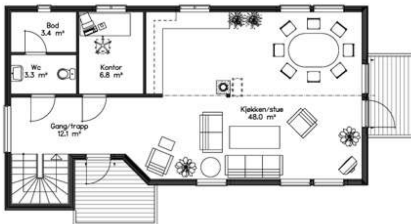
Plan 2. etasje
