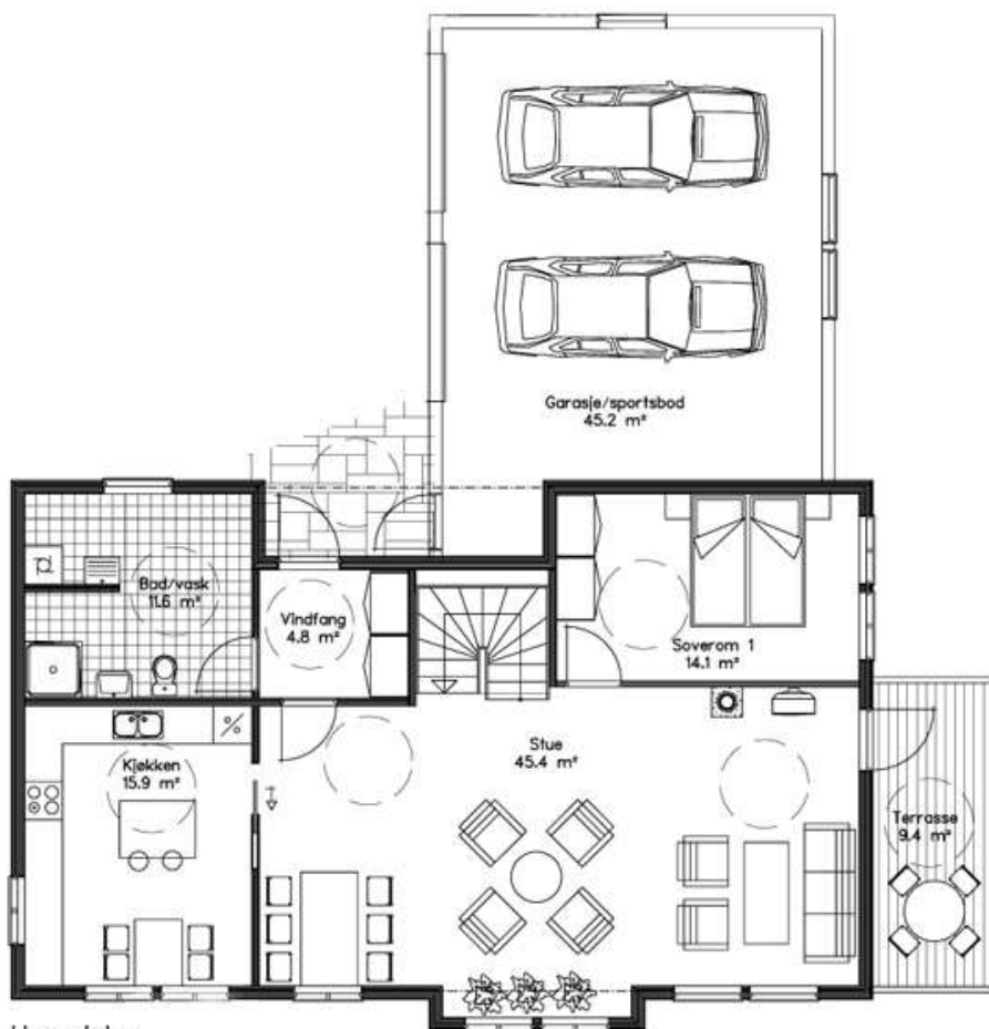
Hovedplan
