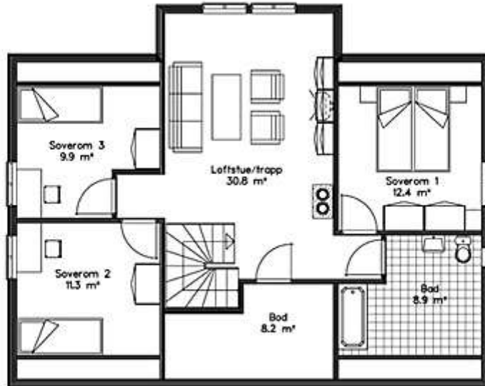
Loftplan
