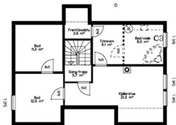
Kjellerplan
